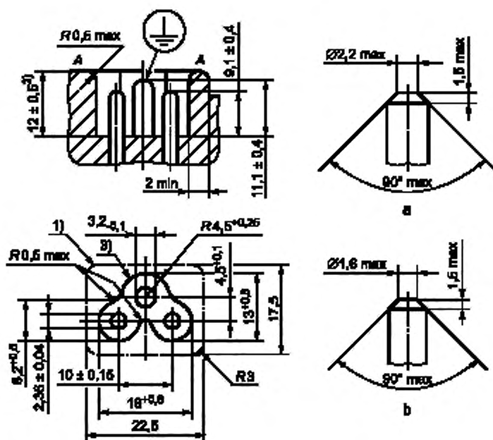
a — заземляющий штырь; b — токопроводящий штырь
