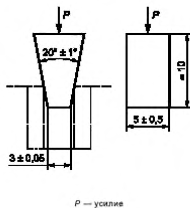
Рисунок 8 — Калибр «непроходной» для розеток по стандартным листам С1 и С7 (ссылка — в 8.4)
