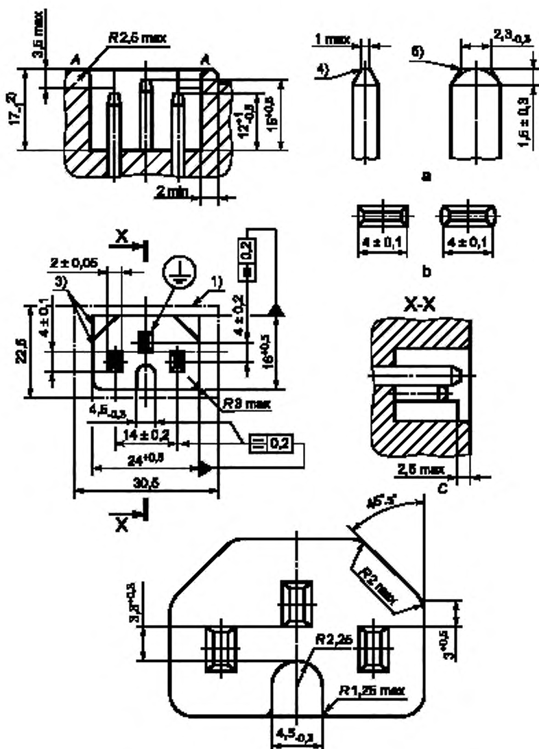
а — вариант исполнения конца штырей; б — варианты формы штырей; с — деталь направляющего элемента
