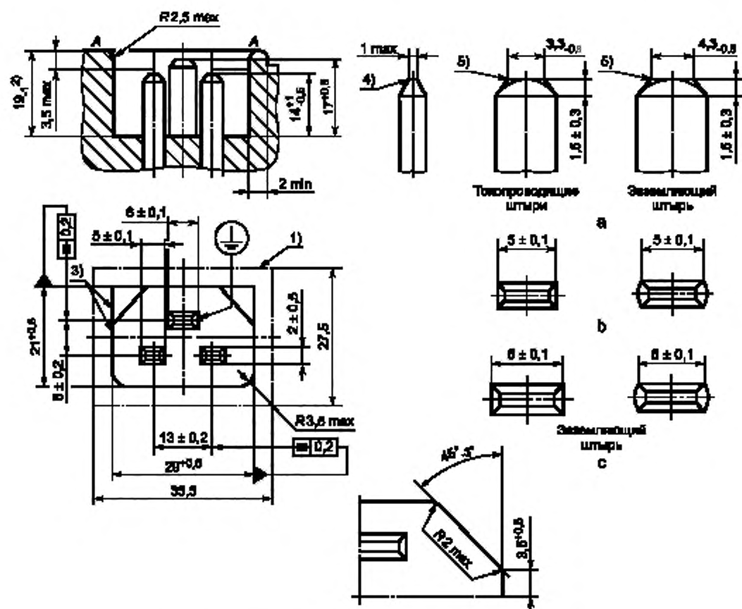
а — вариант исполнения концов штырей; б — варианты формы штырей; в — токопроводящие штыри
