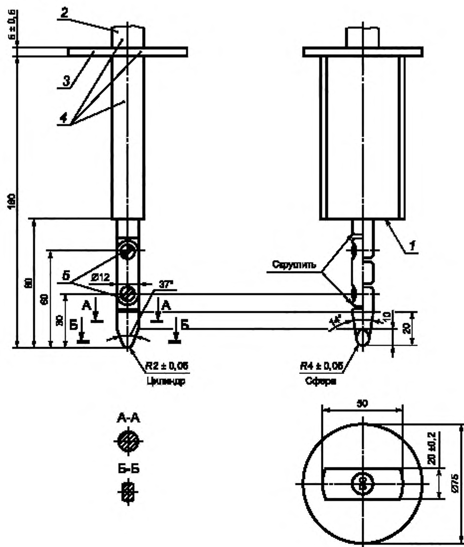
1 — упор; 2 — рукоятка; 3 — упорная пластинка; 4 — изоляционный материал; 5 — шарниры
