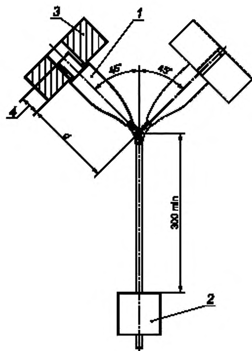
1 — образец; 2 — груз (масса); 3 — деталь качающейся части, на которой закреплён образец; 4 — высота юбки розетки
