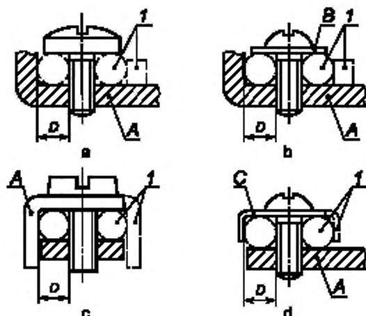
Зажимы с проталкивающей гайкой
