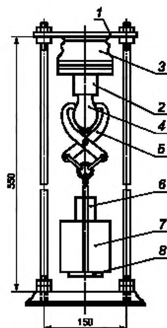
1 — опора; 2 — соединительная вилка; 3 — нагревательное устройство; 4 — образец; 5 — зажим; 6 — дополнительный груз; 7 — основной груз; 8 — пластина
