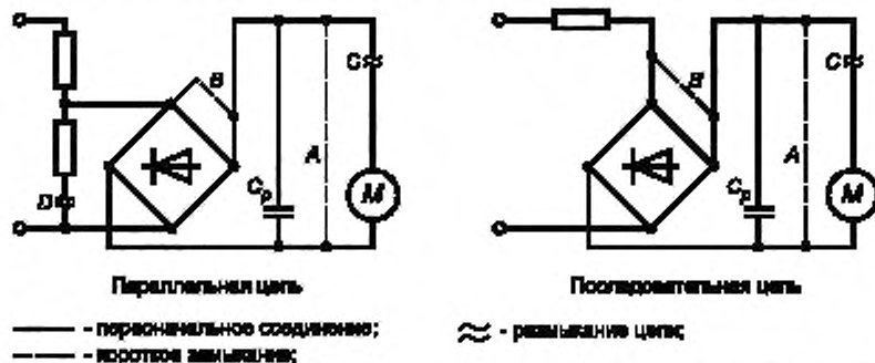
Рисунок 1.1 – Имитация условий неисправности
