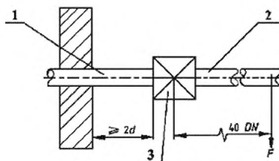
d – внешний диаметр трубы 1 – первая труба; 2 – вторая труба; 3 – испытуемый регулятор Рисунок 1 – Сборочный узел для испытаний регуляторов крутящим моментом
