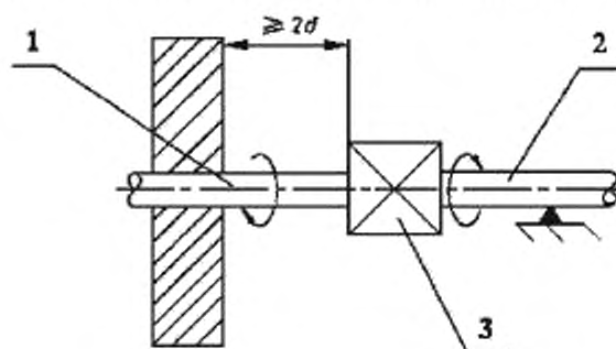
d – внешний диаметр трубы 1 – первая труба; 2 – вторая труба; 3 – испытуемый регулятор Рисунок 2 – Сборочный узел для испытаний регуляторов изгибающим моментом
