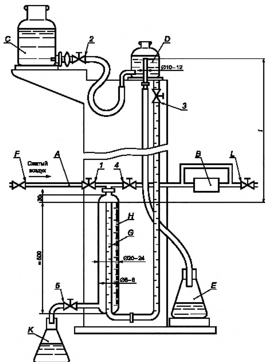
А — вход; В — испытуемый образец; С — емкость с водой; D — сосуд с постоянным уровнем воды; Е, К — переливные сосуды; F — регулятор; G — трубка; H — измерительная бюретка; L — клапан выхода; 1—5 — ручные краны
