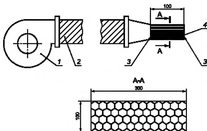
1 — центробежный вентилятор (колесо диаметром 165 мм, электродвигатель мощностью 125 кВт); 2 — гибкий трубопровод; 3 — сетка из проволоки диаметром 0,25 мм с отверстиями диаметром 0,5 мм; 4 — соты с отверстиями размером 5 мм
