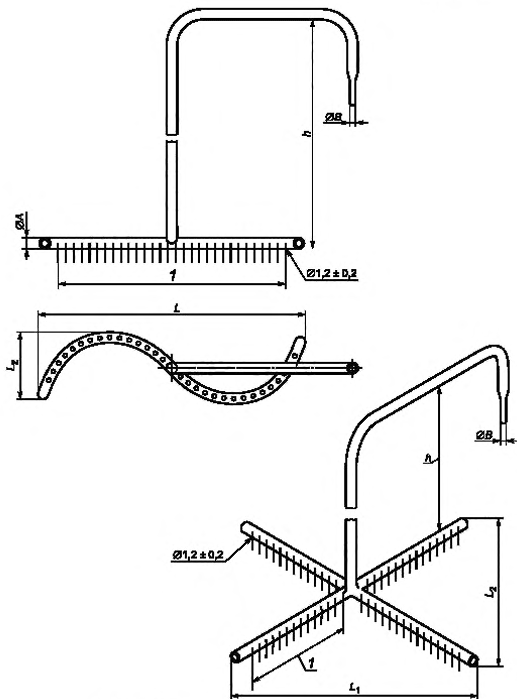
Рисунок 6 — Зонд отбора проб для газовых аппаратов типов А и В с дымовой трубой
