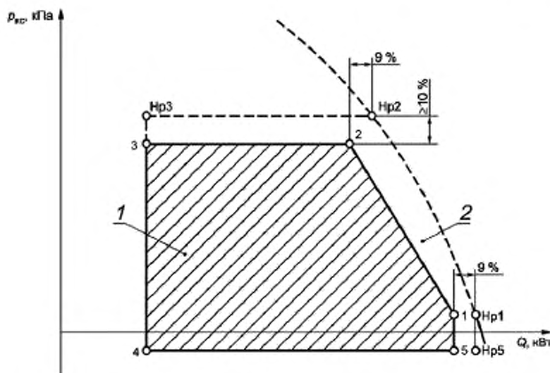
1 — рабочая диаграмма; 2 — испытательная диаграмма
