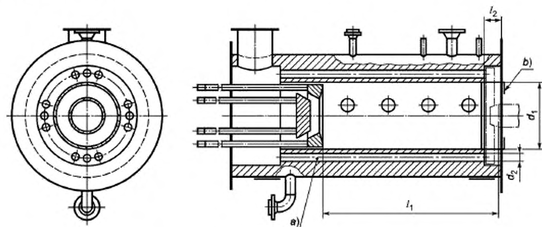
а) — канал рециркуляции продуктов сгорания; б) — регулятор рециркуляции продуктов сгорания (стальной цилиндр)
