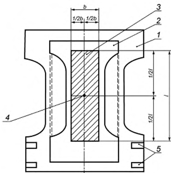
1 — подузник; 2 — первый впитывающий слой подузника; 3 — второй впитывающий слой; 4 — центр второго впитывающего слоя; 5 — застежки-клипчики; l — длина второго впитывающего слоя; b — ширина второго впитывающего слоя
