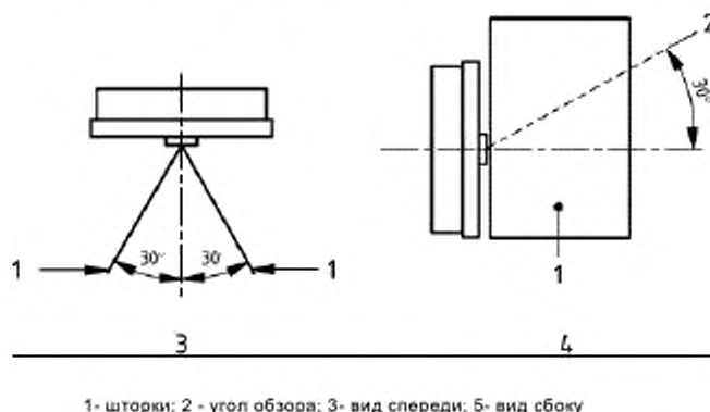
Рисунок 2 — Схематическое представление процесса испытаний на визуальное считывание кода, вид спереди и вид сбоку
