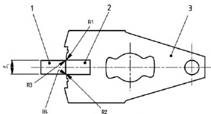
1 – стопорный элемент; 2 – кодовый канал; 3 – сужающая
