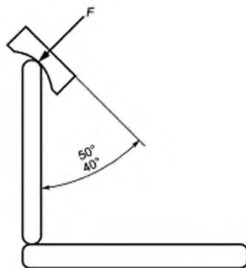
Рисунок 18 — Пример приложения силы сзади к опоре спины
