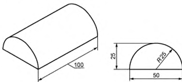
Рисунок 9 — Пример выпуклой нагрузочной подушки
