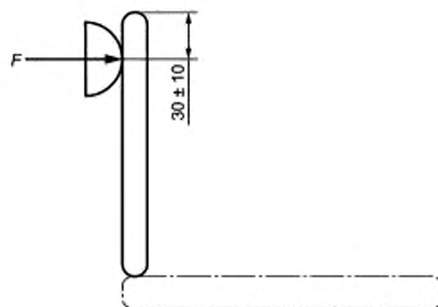
Рисунок 19 — Пример приложения силы спереди к опоре спины
