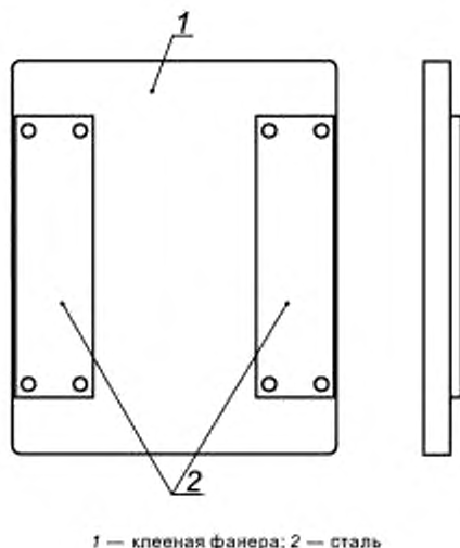
Рисунок 5 — Пример жесткой суррогатной опорной поверхности для испытуемого подсоединяемого приспособления
