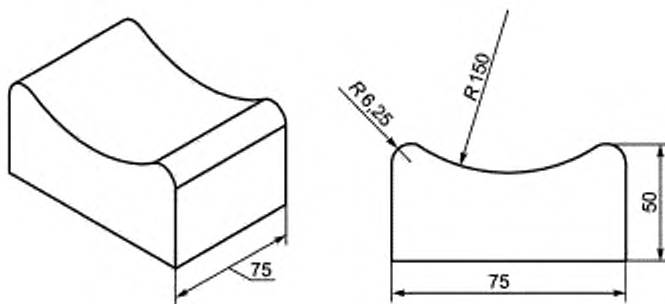
Рисунок 10 — Пример вогнутой нагрузочной подушки
