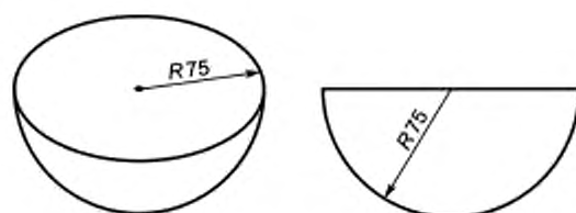
Рисунок 11 — Пример вогнутой полусферической нагрузочной подушки
