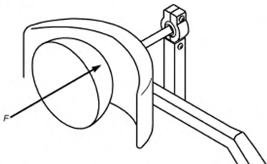
Рисунок 17 — Пример приложения задней силы к опоре головы
