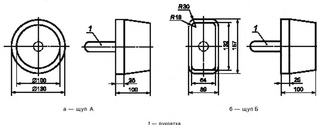
Рисунок Г.1 — Малые щупы для определения застревания головы или шеи ребенка в отверстиях
