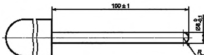
Рисунок Г.12 — Стержень-палец А (малый)
