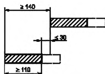
Рисунок 17 — Проекция и глубина ступени
