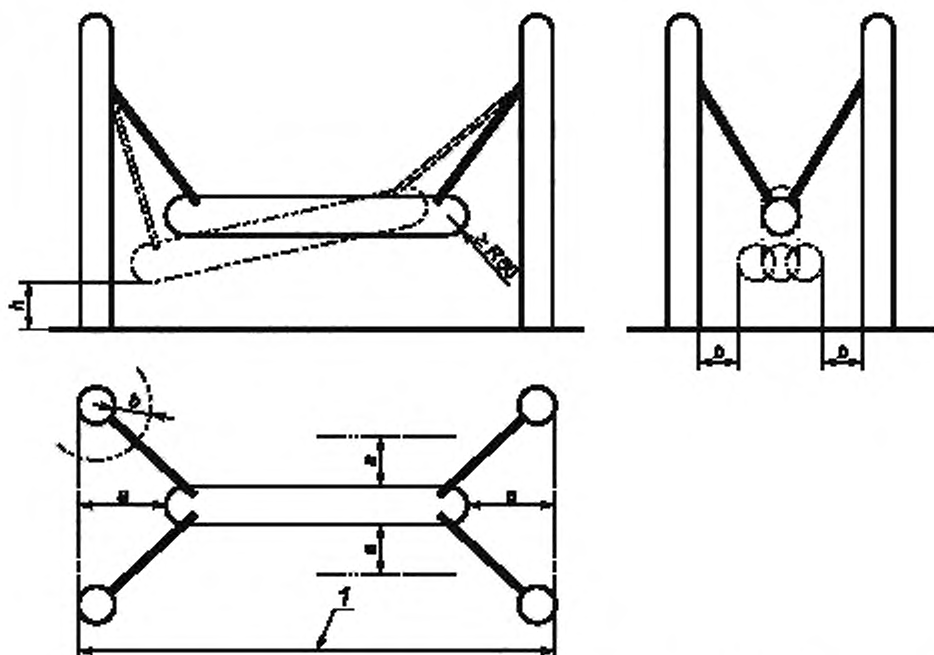
h — расстояние между брусом и поверхностью игровой площадки; a — максимальное горизонтальное и поперечное перемещение бруса; b — расстояние от бруса до опор, l — диапазон перемещения бруса
