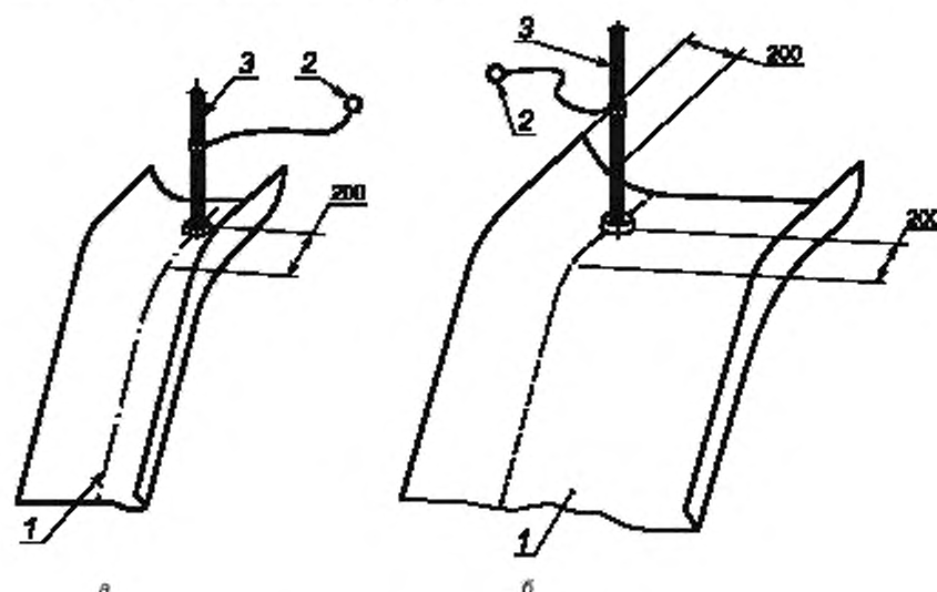
1 — горка; 2 — пуговица с цепью; 3 — стойка
