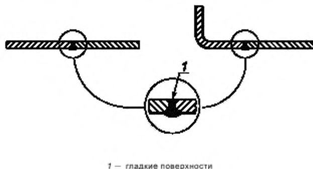
Рисунок А.1 — Гладкие поверхности в пищевой зоне
