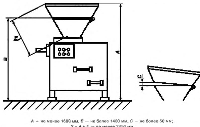
Рисунок 20 — Машины с питающим бункером с разделяющейся воронкой. Безопасные расстояния
