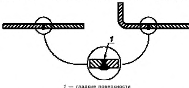
Рисунок А.1 — Гладкие поверхности в пищевой зоне
