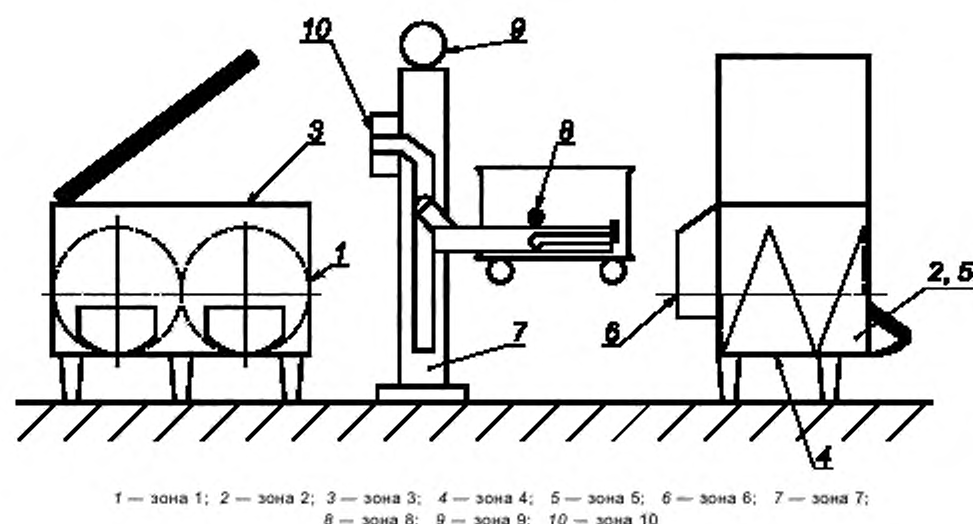
Рисунок 5 — Опасные зоны фаршемешалки
