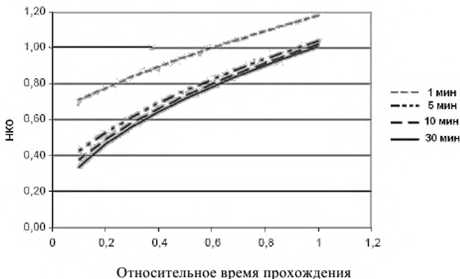
Рисунок Е.7 – Графический пример соотношения между эквивалентным НКО и параметрами при повторно–кратковременном режиме t_1 = 0,5 с, I_1 = 7 \times I_2 для разного времени цикла.
