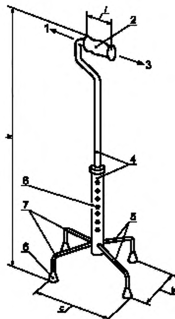
1 — направление движения вперед; 2 — рукоятка; 3 — направление движения назад; 4 — телескопические части; 5 — задние ножки; 6 — наконечник; 7 — передние ножки; 8 — устройство регулировки и фиксации высоты; l — длина рукоятки; b — габаритная ширина трости; c — габаритная длина трости по горизонтали; h — высота трости
