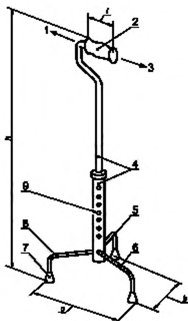
1 — направление движения вперед; 2 — рукоятка; 3 — направление движения назад; 4 — телескопические части; 5 — боковая ножка; 6 — задняя ножка; 7 — наконечник; 8 — передняя ножка; 9 — устройство регулировки и фиксации высоты; l — длина рукоятки; b — габаритная ширина трости; c — габаритная длина трости по горизонтали; h — высота трости
