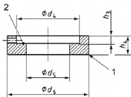
1 – фаска; 2 – углубление (размеры: 1,6 × 0,3 мм)
