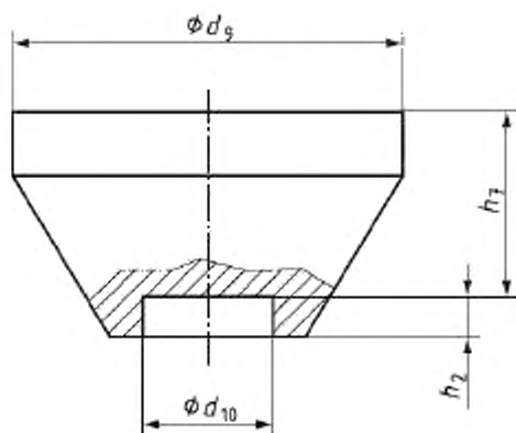
б) нагрузочная опора, уменьшающая поверхностное давление для датчиков силы, имеющих выпуклую поверхность приложения силы
