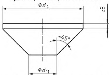
б) нагрузочная опора, уменьшающая поверхностное давление для датчиков силы, имеющих плоскую поверхность приложения силы
