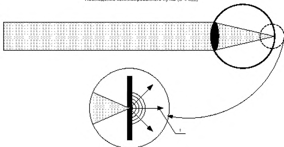
Наблюдение коллимированного пучка ( \alpha < \alpha_{\min} )
