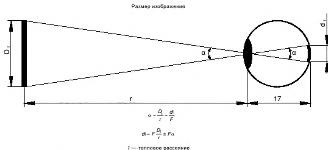
Рисунок 4 — Стыгиваемый угол, охлаждение сетчатки глаза и размер изображения для длин волн в опасной для сетчатки области
