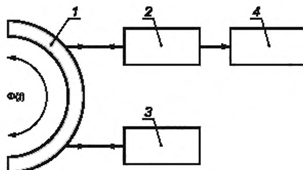
1 — дифракционная решетка; 2 — интерферометр; 3 — калибруемый лазерный виброметр; 4 — система обработки сигнала
