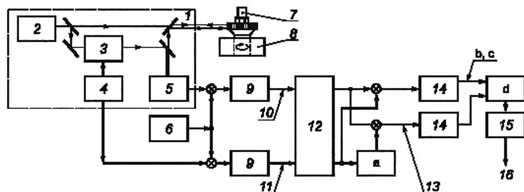
1 — интерферометр, 2 — лазер, 3 — камера Брегга; 4 — кварцевый генератор; 5 — фотодетектор; 6 — синтезирующий генератор, 7 — калибруемый акселерометр; 8 — вибростенд с воздушной подушкой; 9 — низкочастотный фильтр; 10 — измерительный сигнал, 11 — опорный сигнал; 12 — регистратор формы сигнала (переходных процессов); 13 — квадратурные сигналы; 14 — цифровая фильтрация; 15 — алгоритмы обработки; 16 — результаты измерения (параметры вибрации и удара); а — фазовращатель (на 90°); б, с — сигналы y(t) , z(t) ; d — преобразование \arctan y(t)/z(t)
