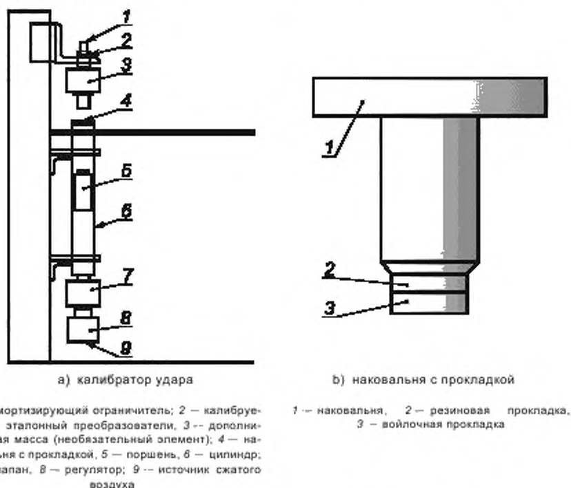
Рисунок 5 — Пример калибратора удара с пневматическим поршнем
