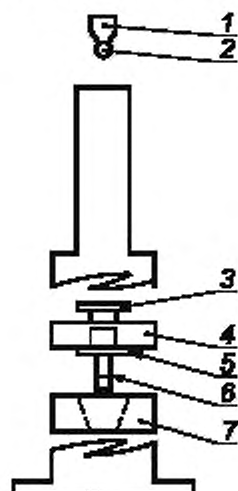
1 — вакуумный держатель; 2 — стальной шар; 3 — плунжер (необязательный элемент); 4 — магнитный держатель; 5 — наковальня; 6 — преобразователи; 7 — улавливающий механизм
