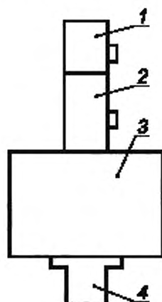
1 — калибруемый преобразователь; 2 — эталонный преобразователь; 3 — сейсмическая масса; 4 — наковальня
