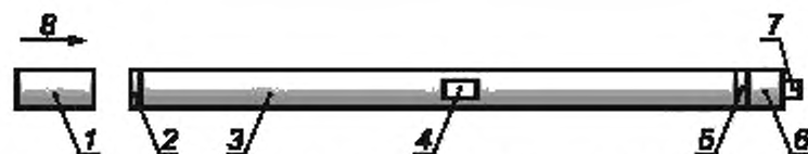
1 — ударник; 2 — формирователь формы импульса; 3 — входной стержень Гопкинсона; 4 — тензометр для получения эталонной кривой; 5 — кварцевая пластина толщиной 0,254 мм; 6 — выходной стержень в виде стального диска длиной 12,7 мм; 7 — калибруемый преобразователь; 8 — начальное движение ударника со скоростью v_0
