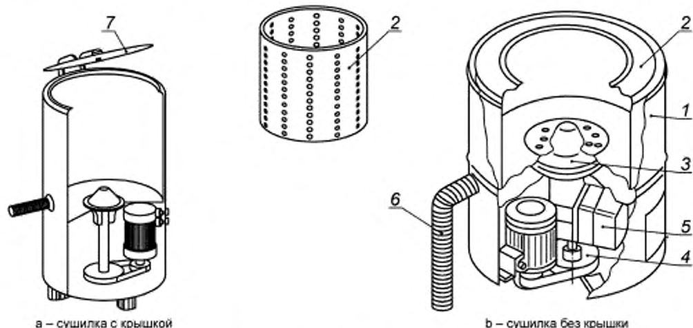
Рисунок 1 — Примеры сушилок
