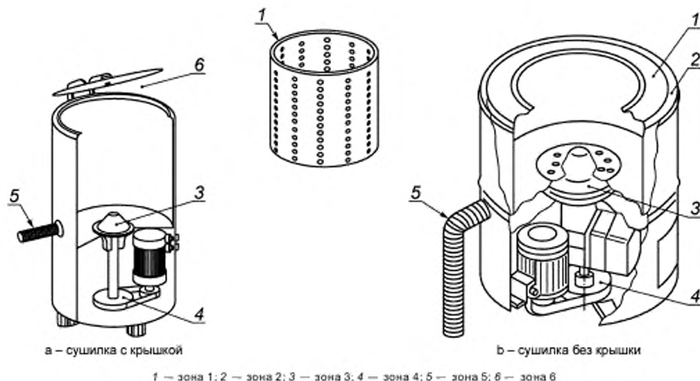
Рисунок 2 — Опасные зоны сушиллки
