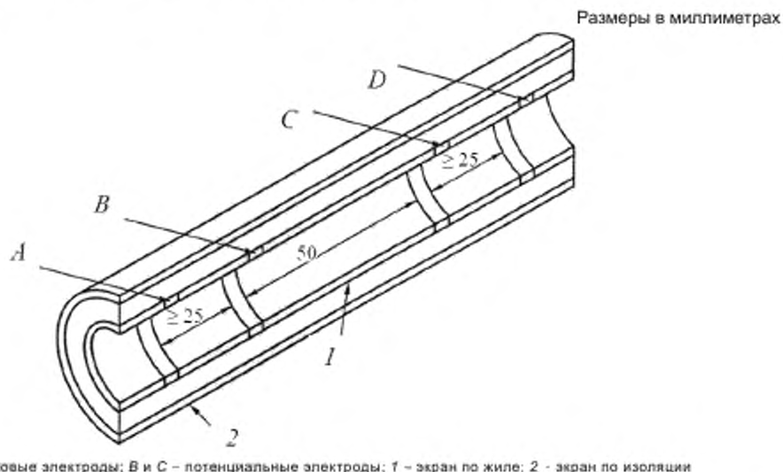
Рисунок Б.1 – Схема измерения электрического сопротивления экструдированного электропроводящего экрана по токопроводящей жиле
