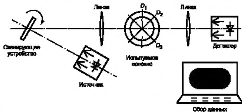
Рисунок A.2 — Оборудование для проведения измерения методом боковой проекции
