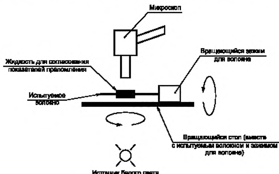
Рисунок А.1 — Типовая испытательная установка
