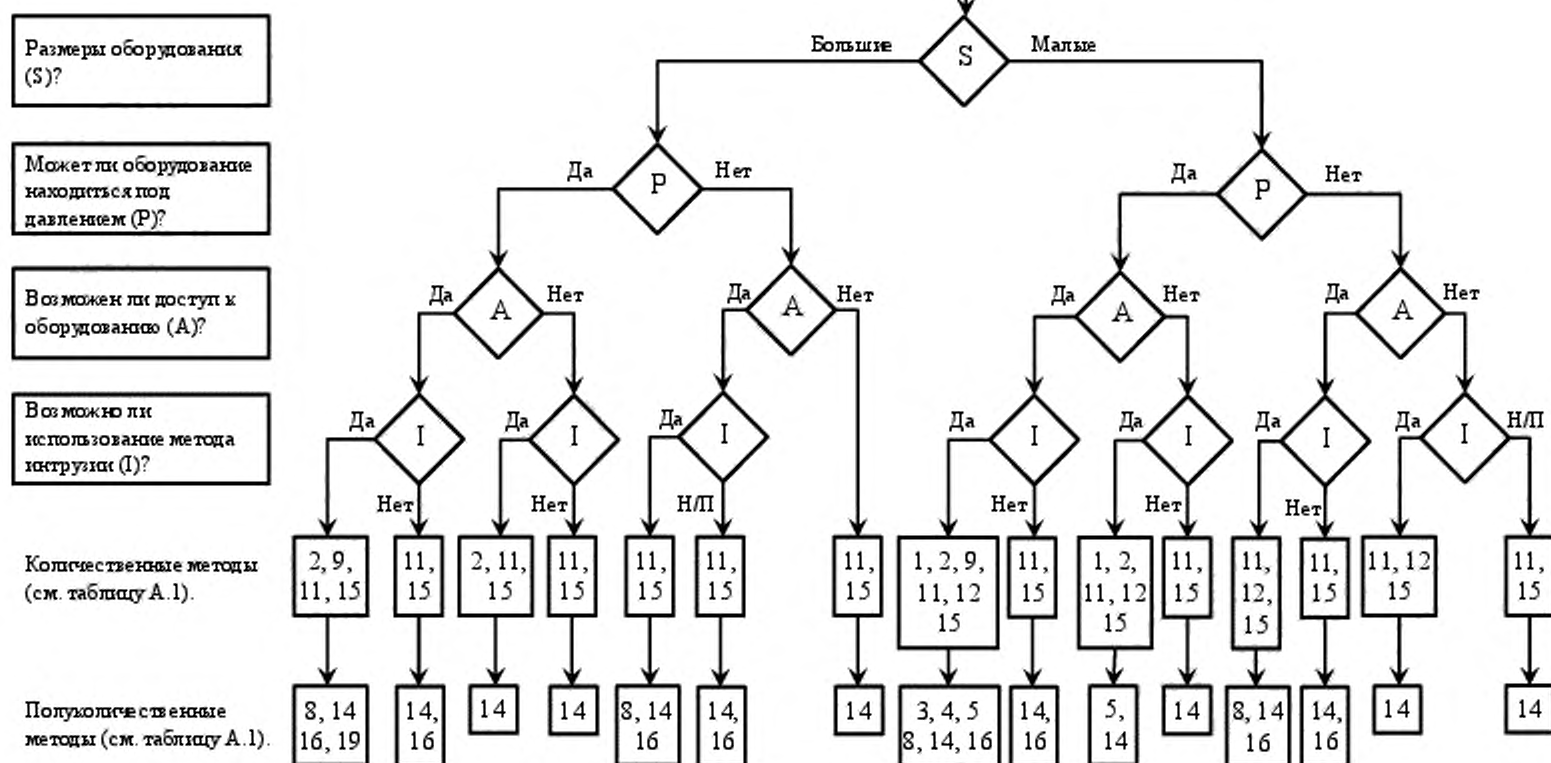
Рисунок А.3 – Дерево решений для выбора метода испытаний на герметичность
