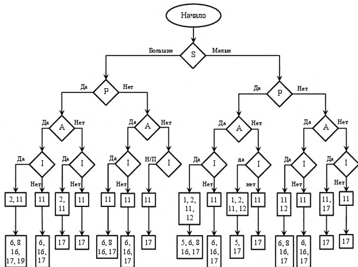
Рисунок А.4 – Дерево решений для выбора метода испытаний на герметичность
