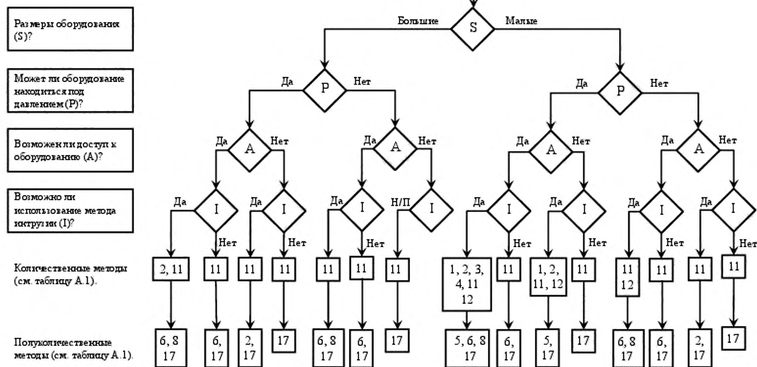
Рисунок А.2 – Дерево решений для выбора метода испытаний на герметичность
