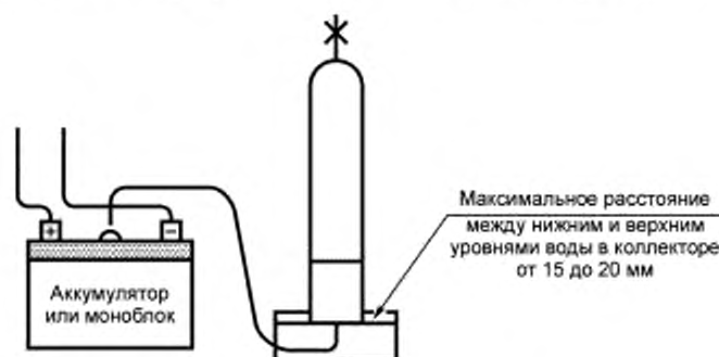
Рисунок 1 — Пример приспособления для сбора газа
