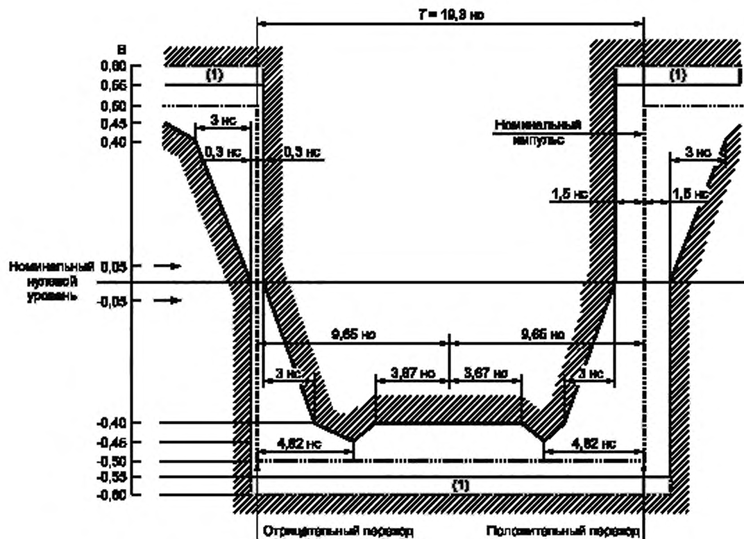
Рисунок Б.2 — Маска импульса 51840 кбит/с 1) 2) (CMI; «1»)
