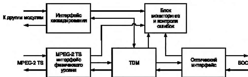
Рисунок 6 — Структурная схема аппаратуры передачи MPEG-2 TS по BOC
