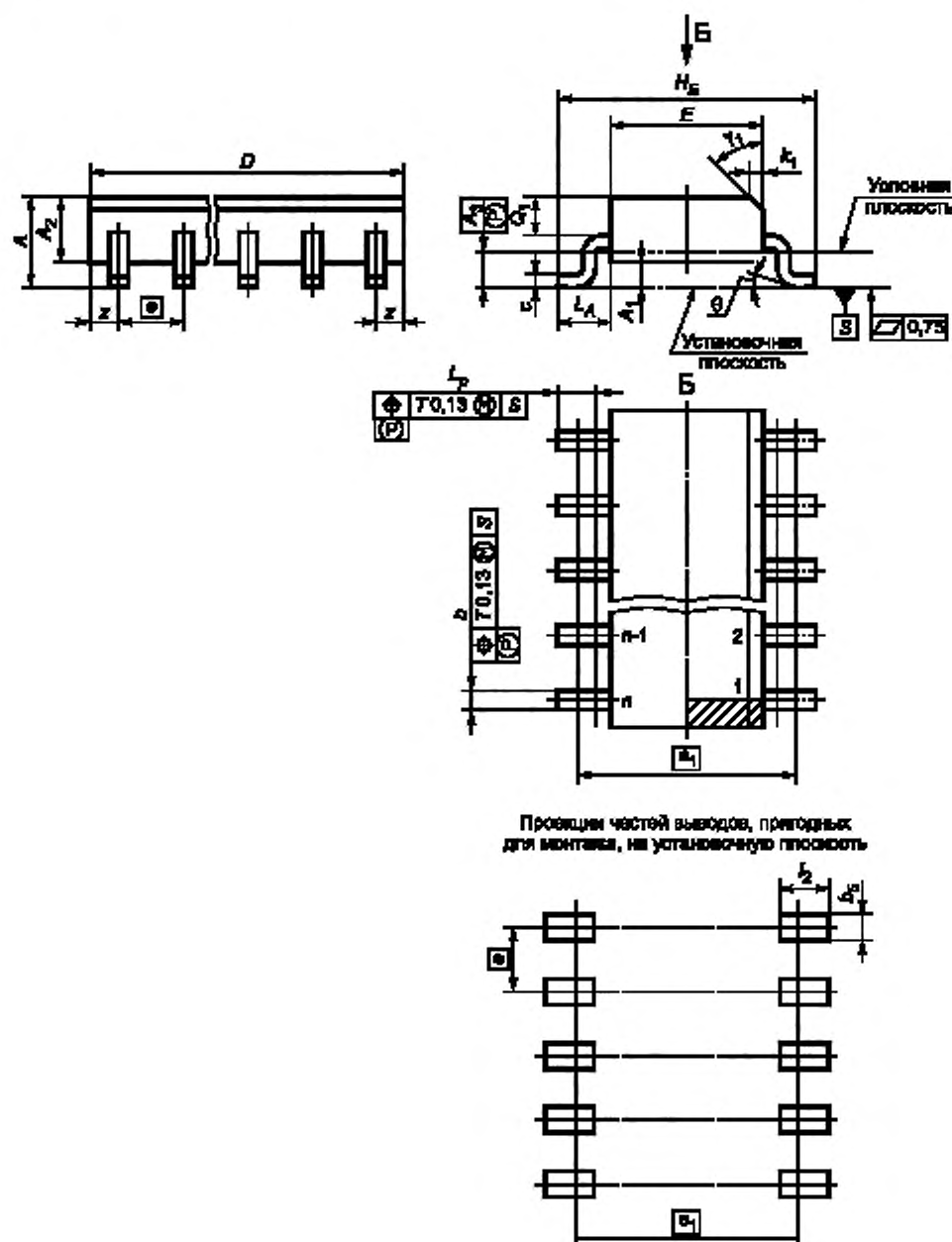
Рисунок 13 — Микросхемы в корпусах подтипа 43
