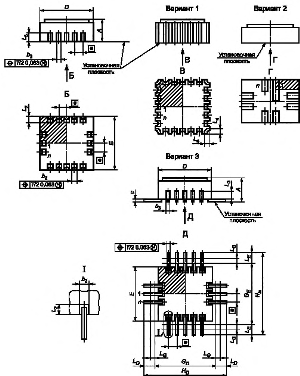
Рисунок 16 — Микросхемы в корпусах подтипа 51
