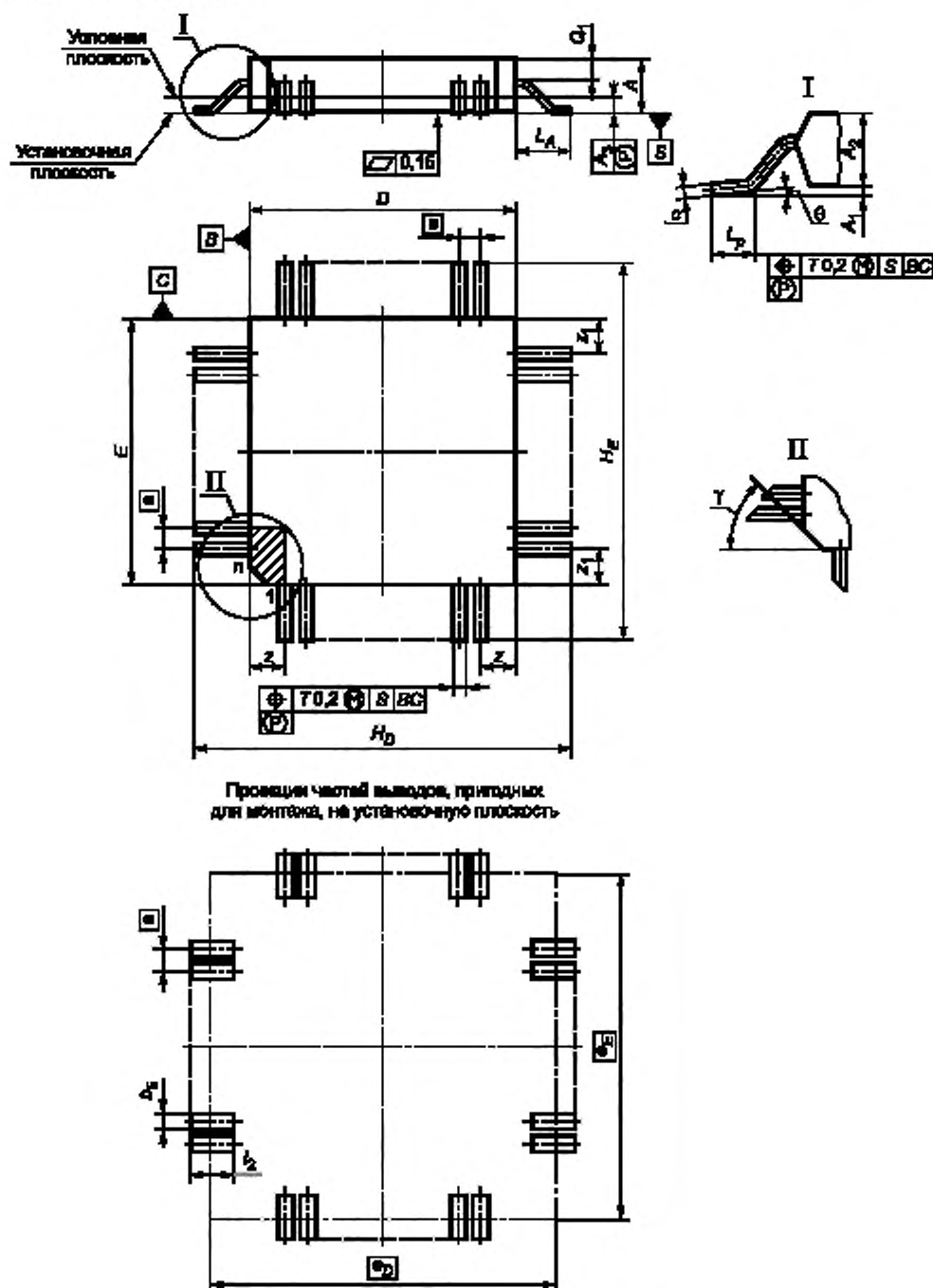
Рисунок 14 — Микросхемы в корпусах подтипа 44
