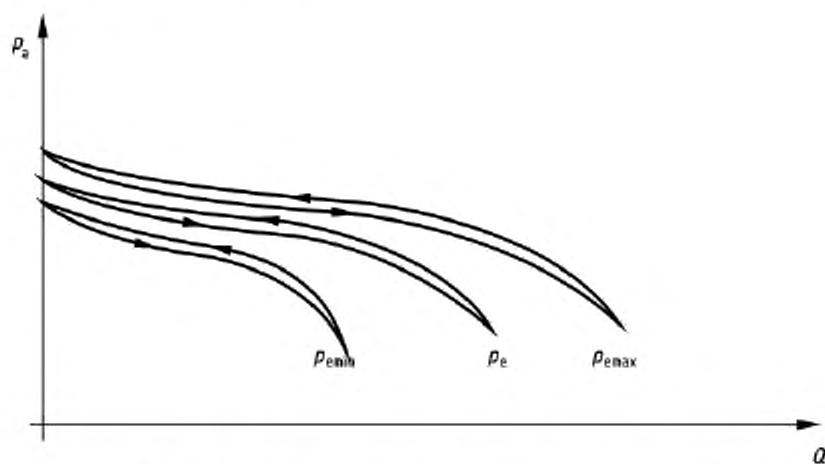
Рисунок 2 — Кривая ( p_{дз} — постоянная, p_{в} — постоянная)
