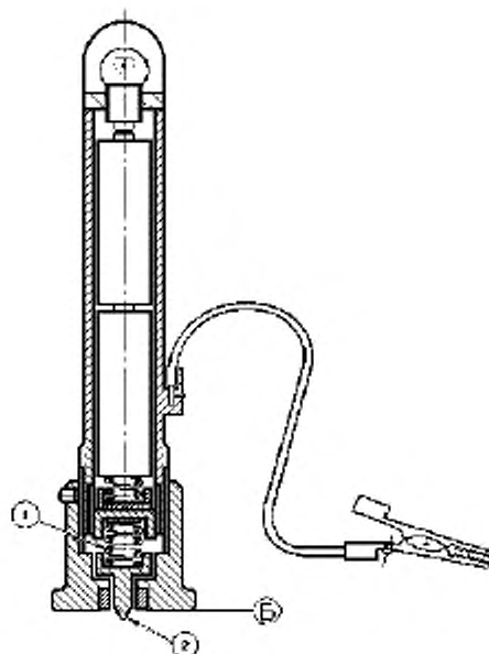
1 — Пружина с усилием 10 Н; 2 — Наконечник, которым проводят испытание царапаньем (стальная сфера диаметром 1 мм)
