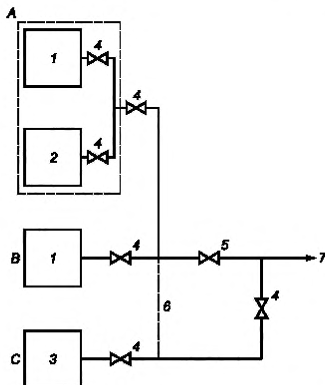
А — первичный источник подачи; В — вторичный источник подачи; С — резервный источник подачи; 1 — блок(и) концентратора кислорода; 2 — баллоны высокого давления, содержащие кислород или воздух обогащенный кислородом, или криогенный сосуд(ы) для жидкости; 3 — две группы баллонов высокого давления; 4 — вентиль источника подачи; 5 — запорный вентиль системы подачи; 6 — необязательное соединение; 7 — к отводящей трубопроводной системе
