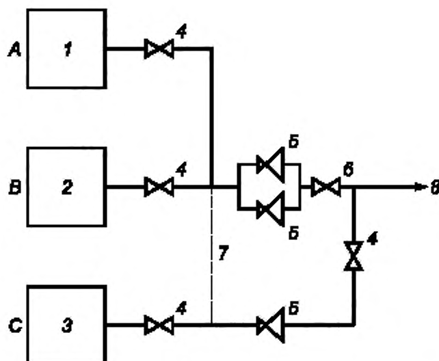
Схематические изображения систем подачи с концентратором кислорода
