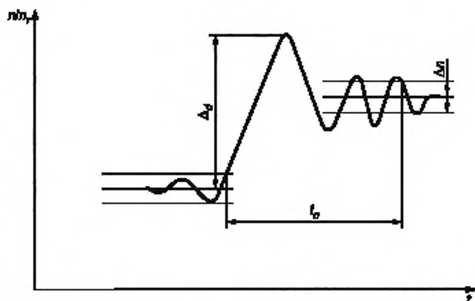
Рисунок 3 — Переходный процесс регулирования после сброса нагрузки
