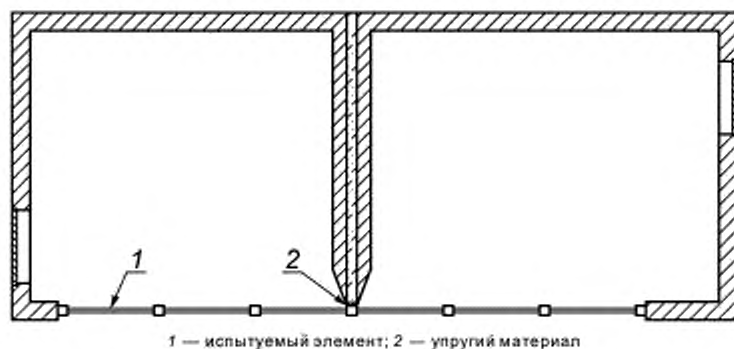
Рисунок 3 — Пример установки фасада. Горизонтальная звукопередача (вид сверху)
