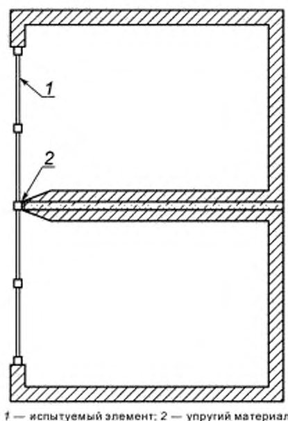
Рисунок 4 — Пример установки фасада. Вертикальная звукопередача (вертикальный разрез)
