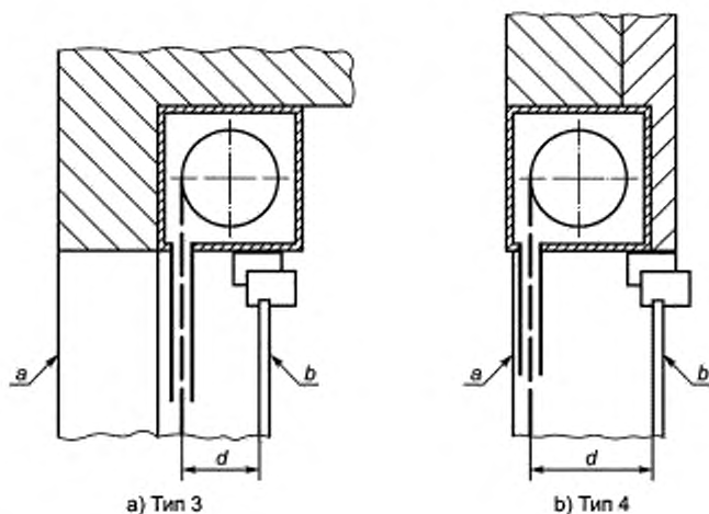
Рисунок 1.2 — Встроенные ставни
