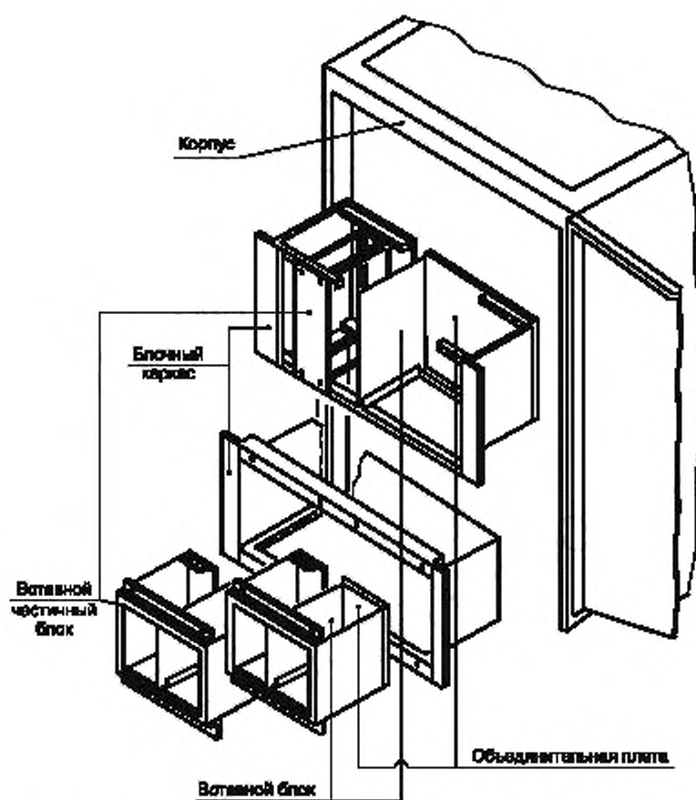
Рисунок 2 — Компоновка вставных блоков, блочных каркасов и корпусов
