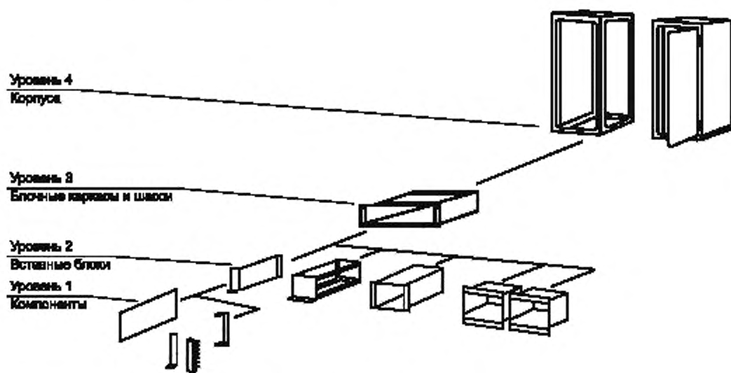
Рисунок 1 — Уровни структуры несущих конструкций*
