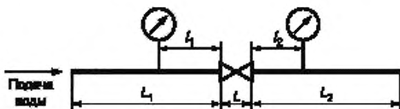
Рисунок 1 — Принципиальная схема участка расходного испытательного стенда
