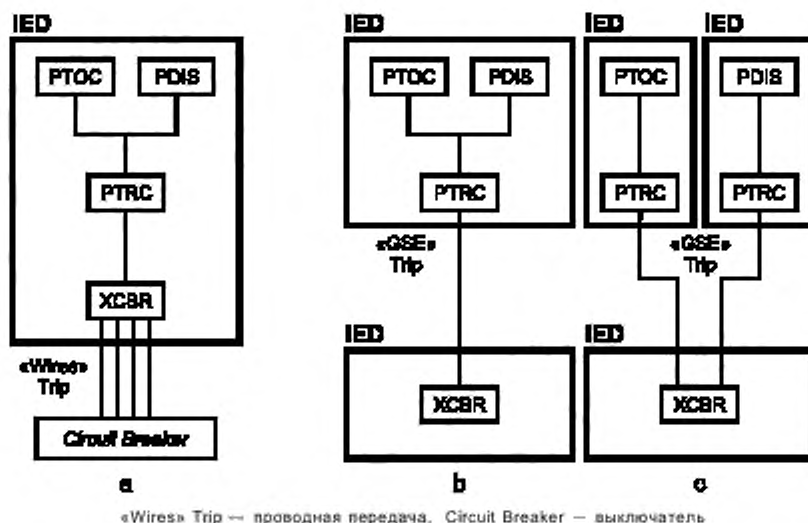
Рисунок B.5 — Пример назначения логических узлов IED-устройствам
