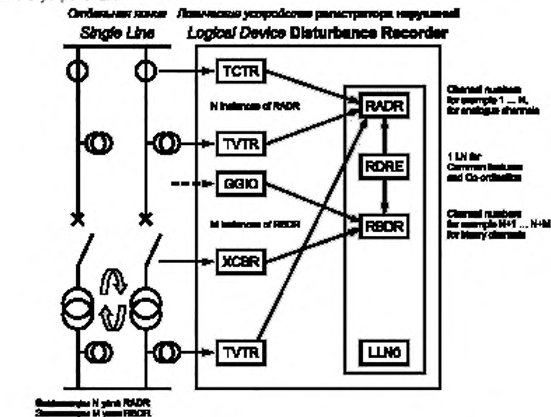
Рисунок В.4 — Моделирование регистратора нарушений
