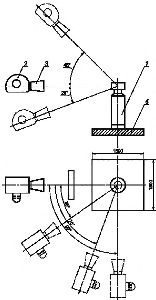
1 — вход воздуха для горения и выпускной канал; 2 — вентилятор; 3 — распылитель; 4 — испытательная поверхность
