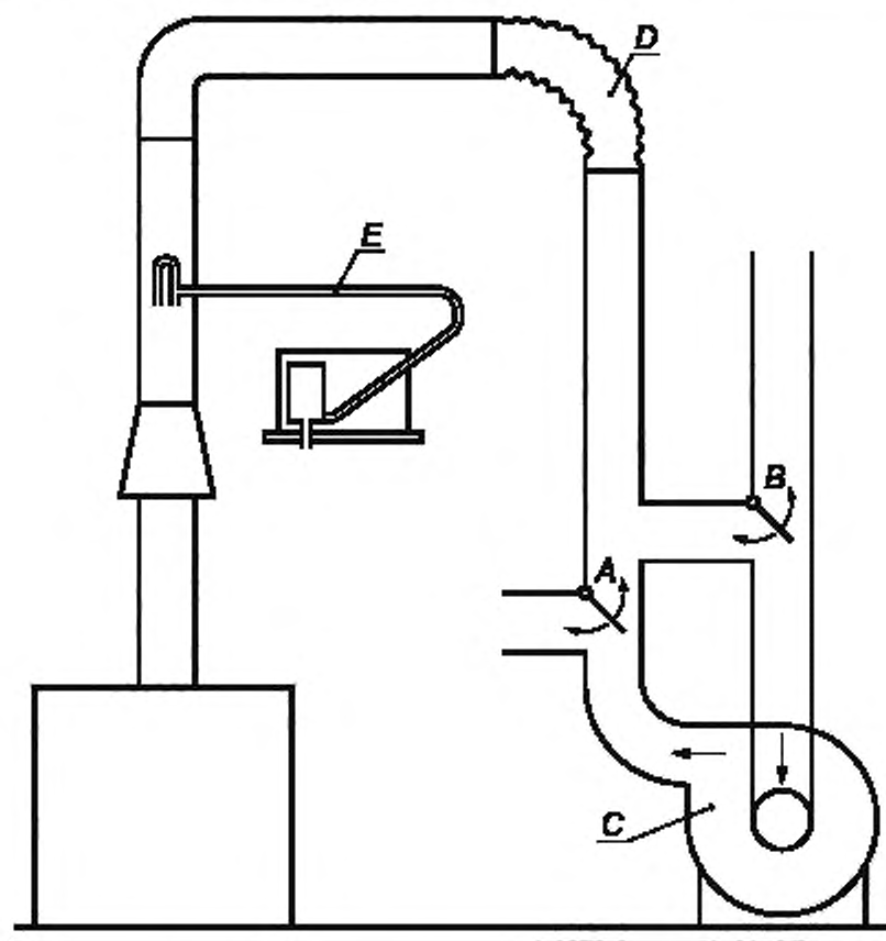
А и В — перегородки для получения восходящей и обратной тяги; С — вентилятор; D — гибкий участок; Е — трубка Пито для измерения скорости потока
