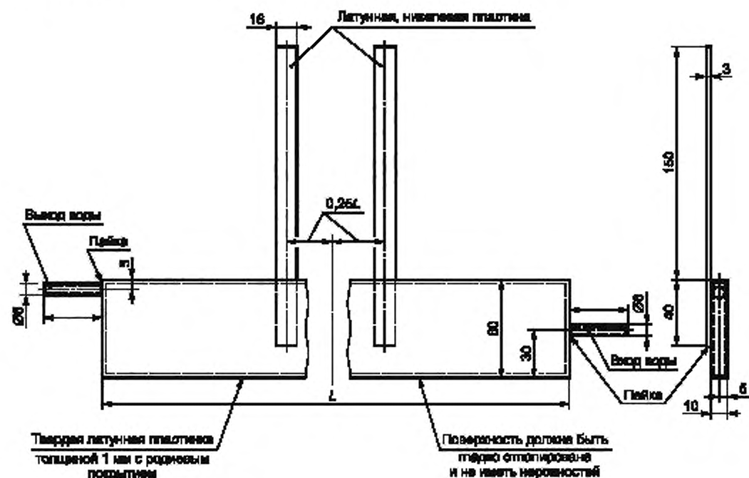
Рисунок 1 — Индикатор утечки (пластинка точки росы)
