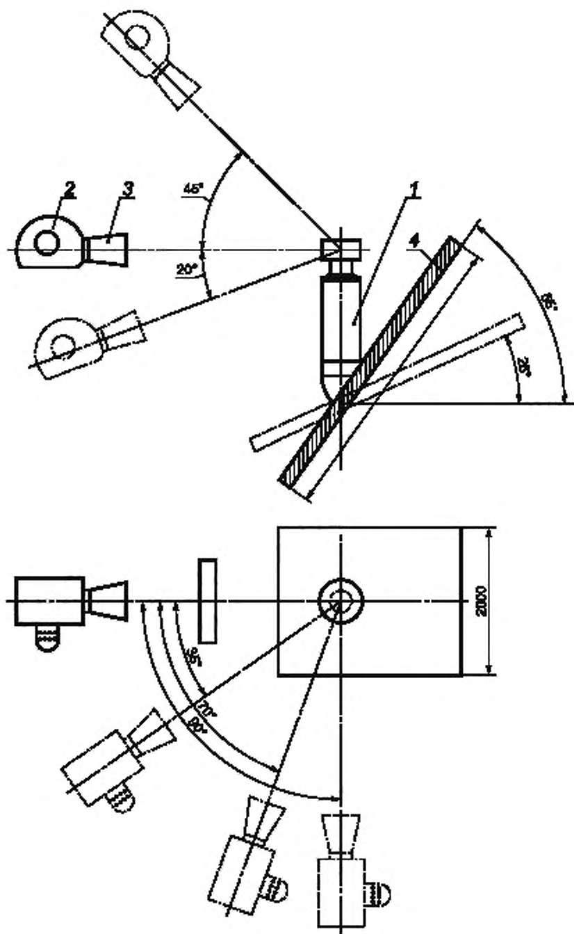
1 — вход воздуха для горения и выпускной канал; 2 — вентилятор; 3 — распылитель; 4 — испытательная поверхность
