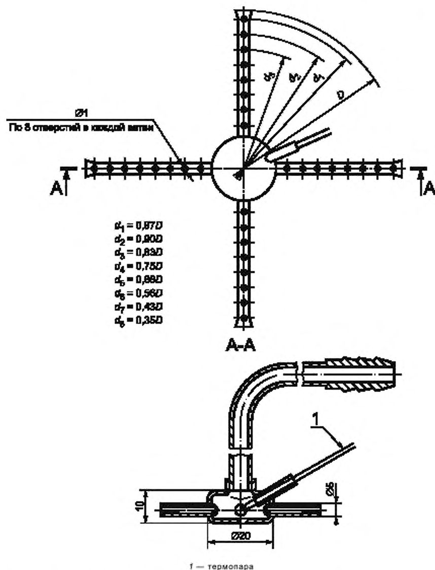
Рисунок 5а — Устройство для отбора проб и измерения температуры продуктов сгорания для дымоходов диаметром D \geq 100 мм (приборы типа В)
