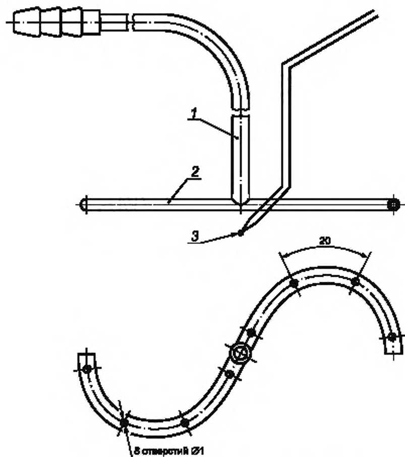
Рисунок 56 — Устройство отбора образцов для приборов типа В. Устройство для отбора проб и измерения температуры продуктов сгорания для дымохода диаметром, не превышающим 100 мм (приборы типа В)
