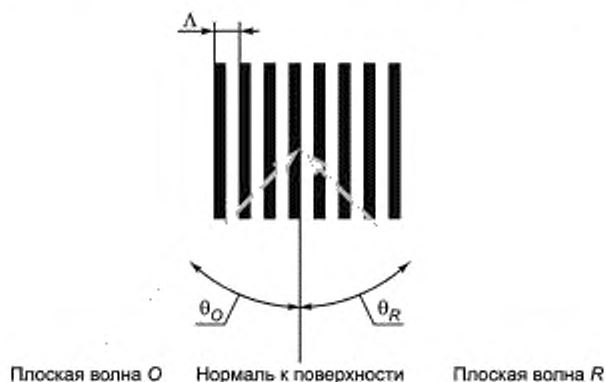
Рисунок А.1 — Запись дифракционной решетки в запоминающем слое при помощи интерференции двух плоских волн
