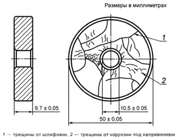
Рисунок В.1 — Эталонный образец типа 1
