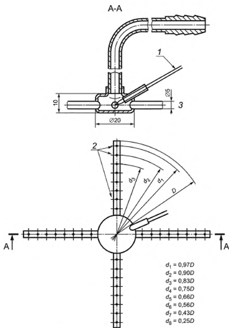
Рисунок 5 — Устройство для отбора проб и измерения температуры продуктов сгорания для дымохода диаметром более 100 мм (см. 7.12.2.1)
