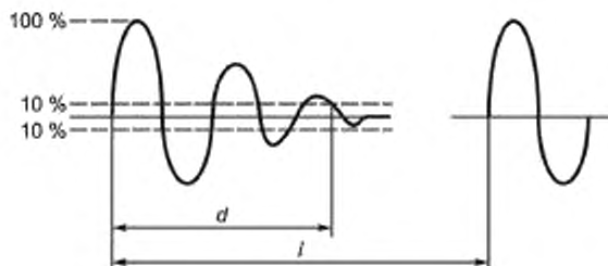
Рисунок G.1 — Кривая напряжения при сопротивлении R
