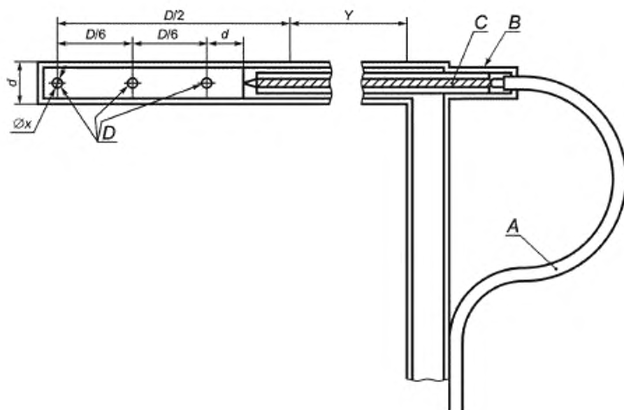
А — провода термопары; В — изолирующий цемент. С — двухканальная керамическая труба, D — три отверстия для отбора проб диаметром x мм
