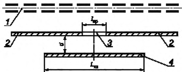
1 — железнодорожный путь; 2 — акустический экран; 3 — проем (разрыв) в акустическом экране; 4 — контрэкранны
