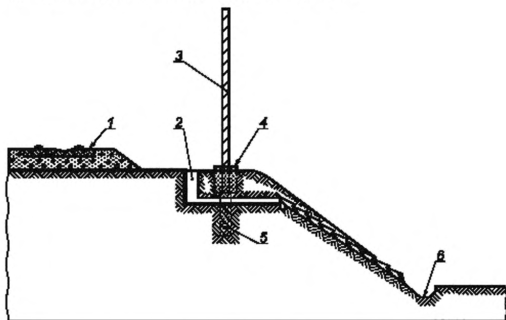
1 — железнодорожный путь, 2 — водосток; 3 — акустический экран; 4 — бетонное основание, 5 — связь для закрепления фундамента АЗ; 6 — лоток для отвода воды
