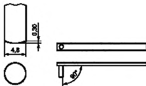
Рисунок В.3 — Пример типичного Г-образного инструмента с углом 90°
