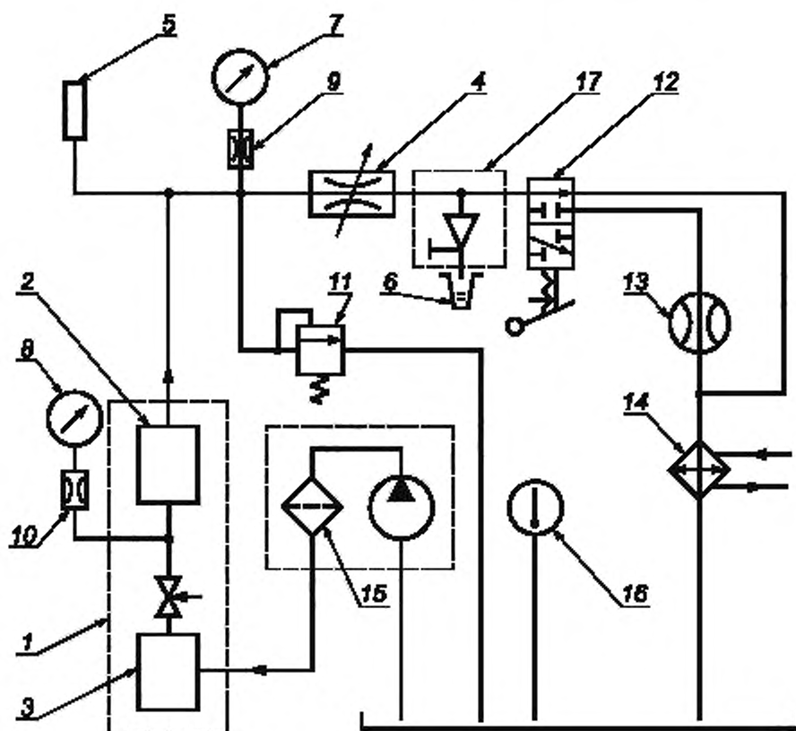
Гидравлическая схема станда для испытаний насосных станций механизированных крепей
