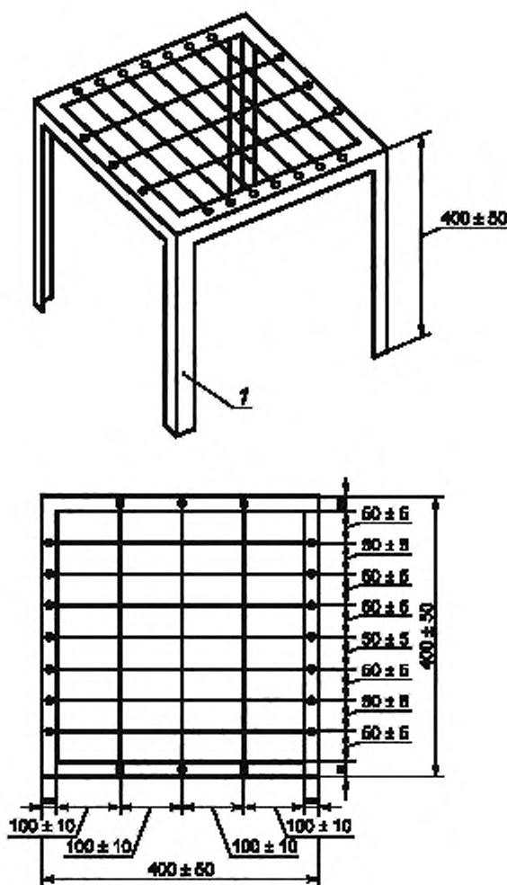
Рисунок 1 — Испытательный стенд
