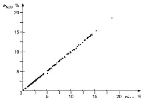
Рисунок F.1 — Зависимость между массовой долей азота, измеренной по методу Дюма и методу Кельдаля для проб, использованных в исследованиях, приведенных в таблице F.1
