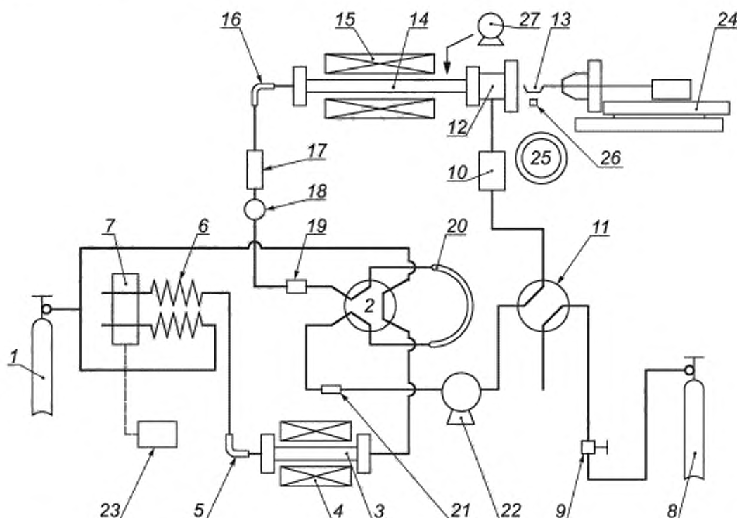
1 — баллон с гелием; 2 — клапан; 3 — восстановительная трубка; 4 — восстановительная печь; 5 — газопоглощающая трубка; 6 — колонка для разделения газов; 7 — детектор теплопроводности; 8 — баллон с кислородом; 9 — регулятор потока кислорода; 10 — расходомер; 11 — клапан; 12 — ввод пробы для анализа; 13 — стержень для ввода пробы для анализа; 14 — трубка-реактор; 15 — печь для нагрева трубки-реактора; 16 — трубка для проверки полноты сгорания; 17 — конденсатор для удаления водяного пара; 18 — трубка для смешивания газов; 19 — фильтр № 1; 20 — измерительная трубка; 21 — фильтр № 2; 22 — циркуляционный насос; 23 — устройство для обработки данных; 24 — устройство для ввода проб для анализа; 25 — лоток для пробы; 26 — подъемное устройство для лотка с пробой; 27 — насос для подачи охлаждающего воздуха
