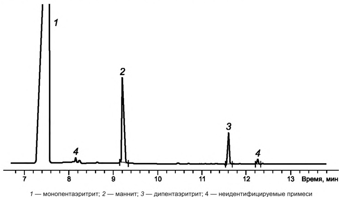
Рисунок 1 — Типовая хроматограмма технического пентаэритрита
