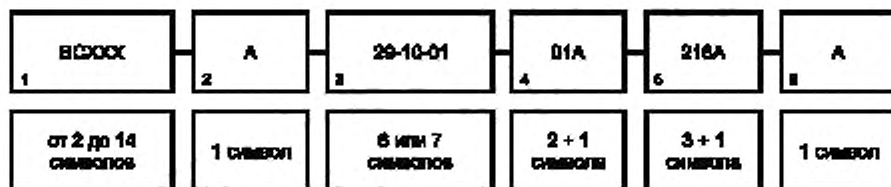
Рисунок 1 — Структура ОМД
