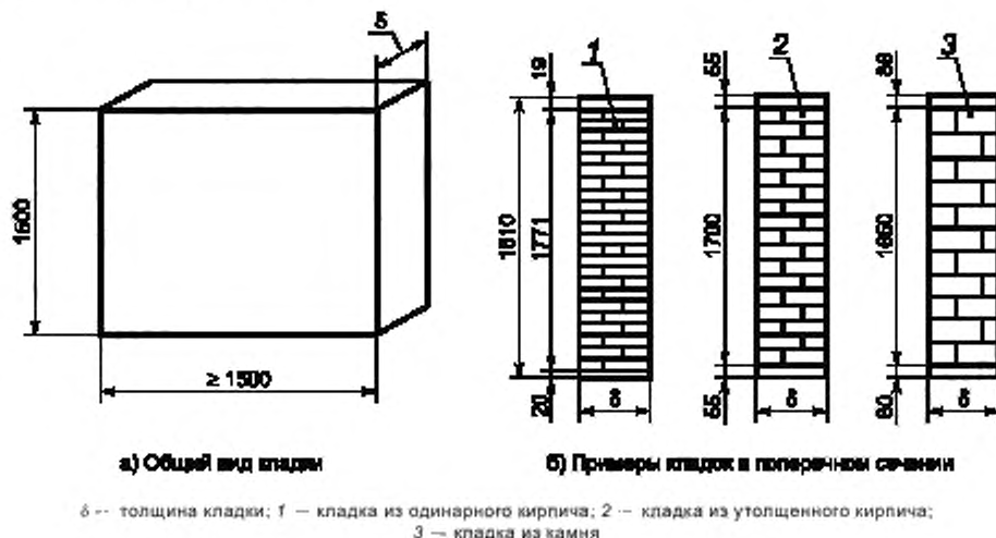
Рисунок 2 — Фрагмент кладки для определения коэффициента теплопроводности
