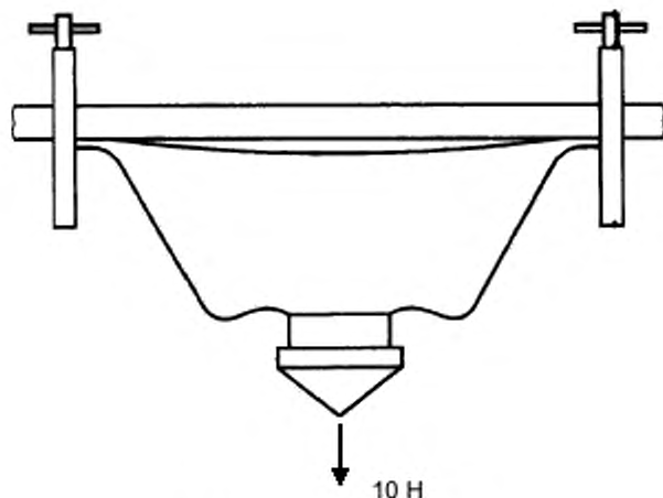
Рисунок 2 – Крепление маски
