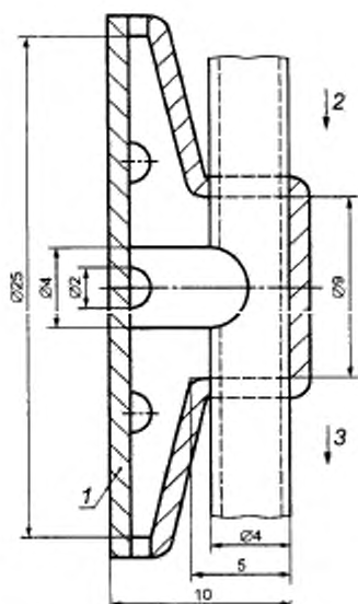
1 – ПВХ; 2 – осушающий воздух; 3 – проба, содержащая осушающий воздух
