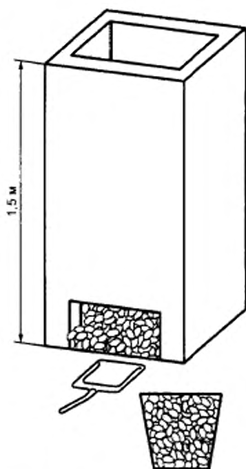
Рисунок 11 — Корзина и контейнер, щебенка
