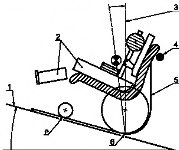
1 — испытательная плоскость; 2 — испытательный манекен; 3 — вертикаль; 4 — ограничитель дальнейшего опрокидывания; 5 — гибкая система удерживания; 6 — ось опрокидывания; P — точка отрыва от испытательной плоскости
