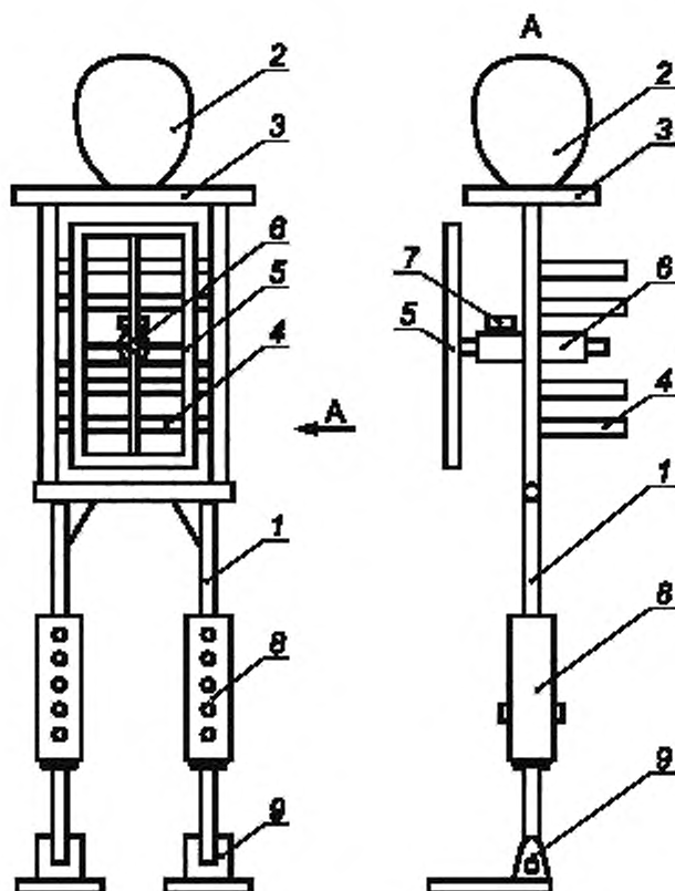
1 — осто́в манекена; 2 — муляж головы человека; 3 — плечево́й каркас; 4 — габаритная скоба; 5 — габаритная ра́мка; 6 — направляющая втулка; 7 — стопорный винт; 8 — регулятор высоты манекена; 9 — подо́шва
