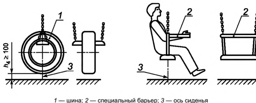
Рисунок 10 — Пример конструкции сидений качелей типа 4
