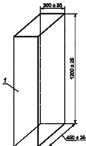
Рисунок 1 — Испытательное оборудование — металлическая камера
